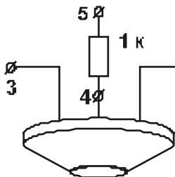
Рис. 4.1. Организация двухполюсного шлейфа пожарной сигнализации
